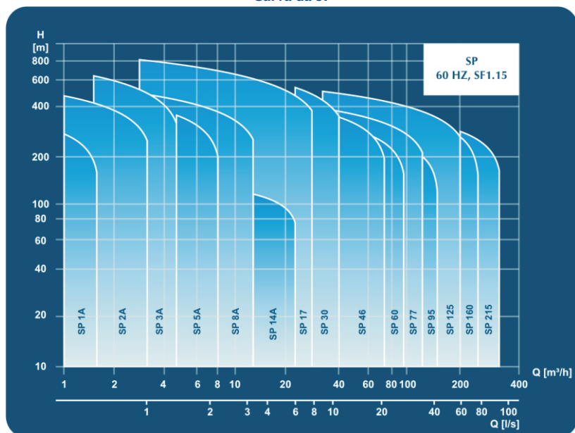
Curva da SP
